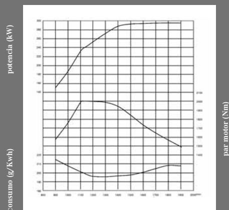
Curvas de desempeño del motor OM-457 LA
